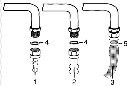
1 Hortum ucu-LPG
